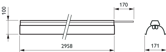
TTX260 4 x TL5 C-NB
