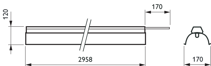
TTX260 2 x TL5 WR
