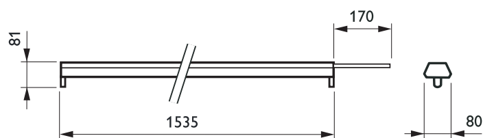
TTX261/262/263 1 x TL-D 58 W
