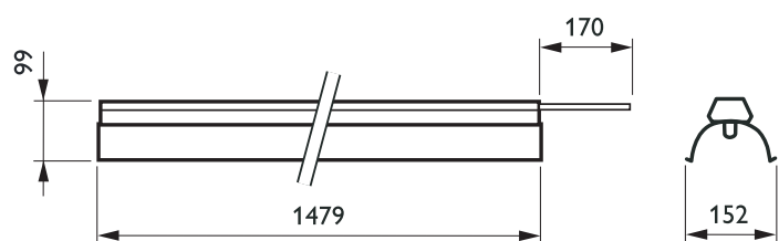
TTX261/262/263 1 x TL5 C-MB
