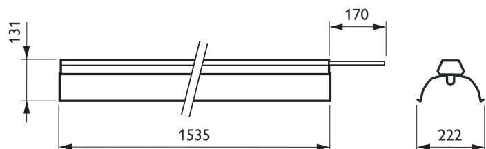
TTX261/262/263 1 x TL-D 58 W WR
