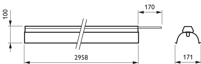
TTX260 2 x TL5 C-NB
