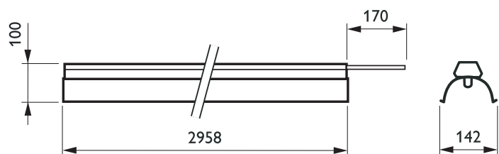
TTX260 2 x TL5 C-WB/CP-WB
