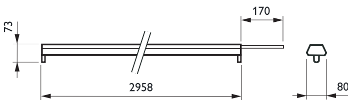
TTX260 2 x TL5
