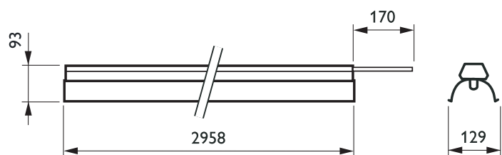
TTX260 2 x TL5 C-DA
