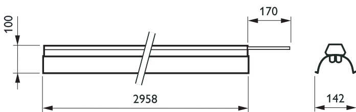
TTX260 4 x TL5 C-WB/CP-WB
