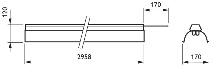
TTX260 4 x TL5 WR
