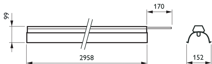
TTX260 2 x TL5 C-MB
